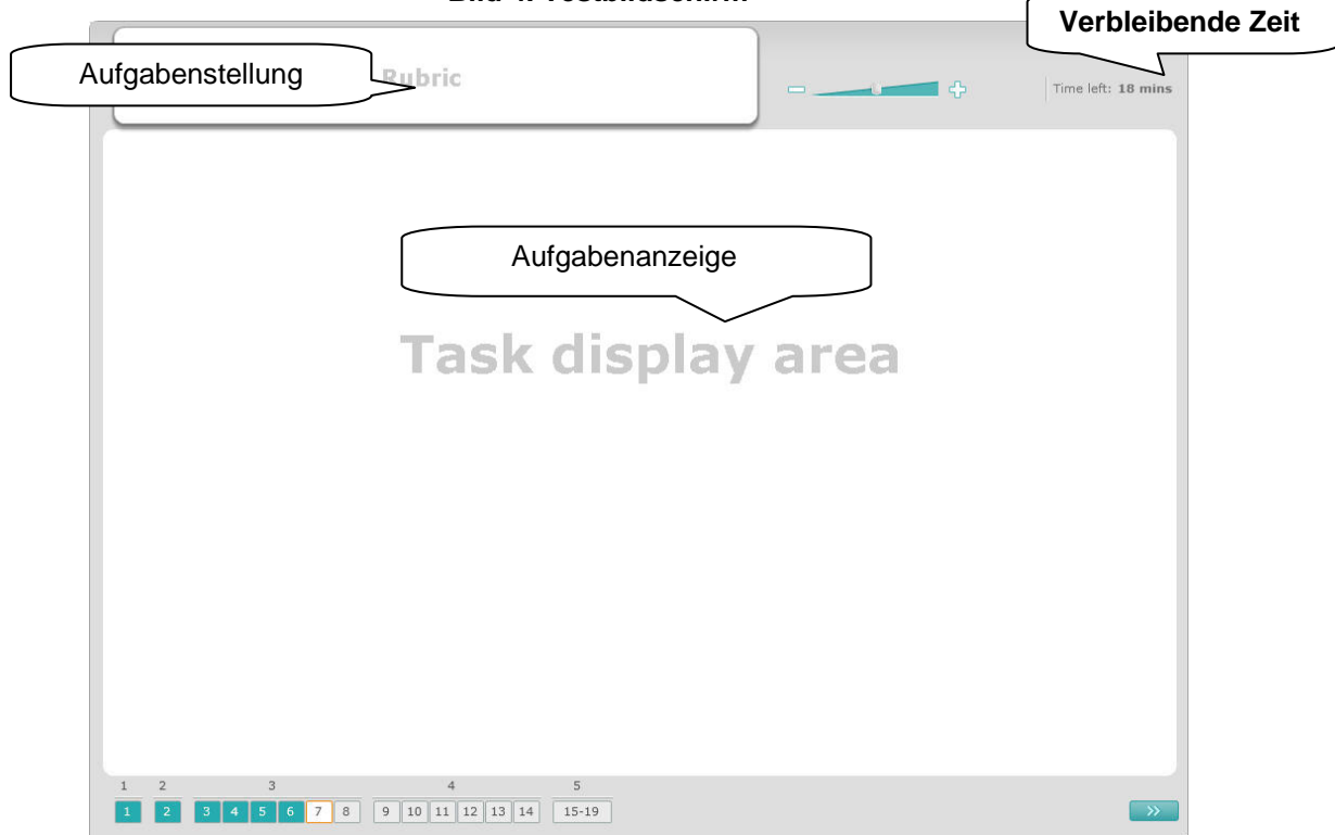
Bild 4. Testbildschirm
